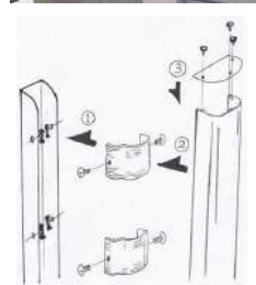
取り付けイメージ
