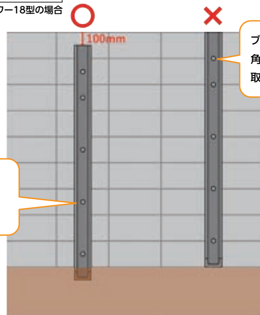
立面図 ※FITパワー18型の場合
