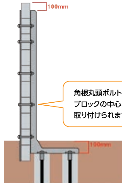
断面図 ※FITパワー18型の場合
